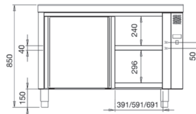
MEDIDAS MESA CALIENTE
