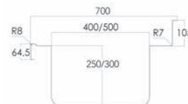
MEDIDAS CUBETA
