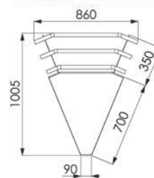
MEDIDAS MODELO S1000412
