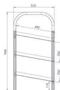
MEDIDAS DISPENSADOR
